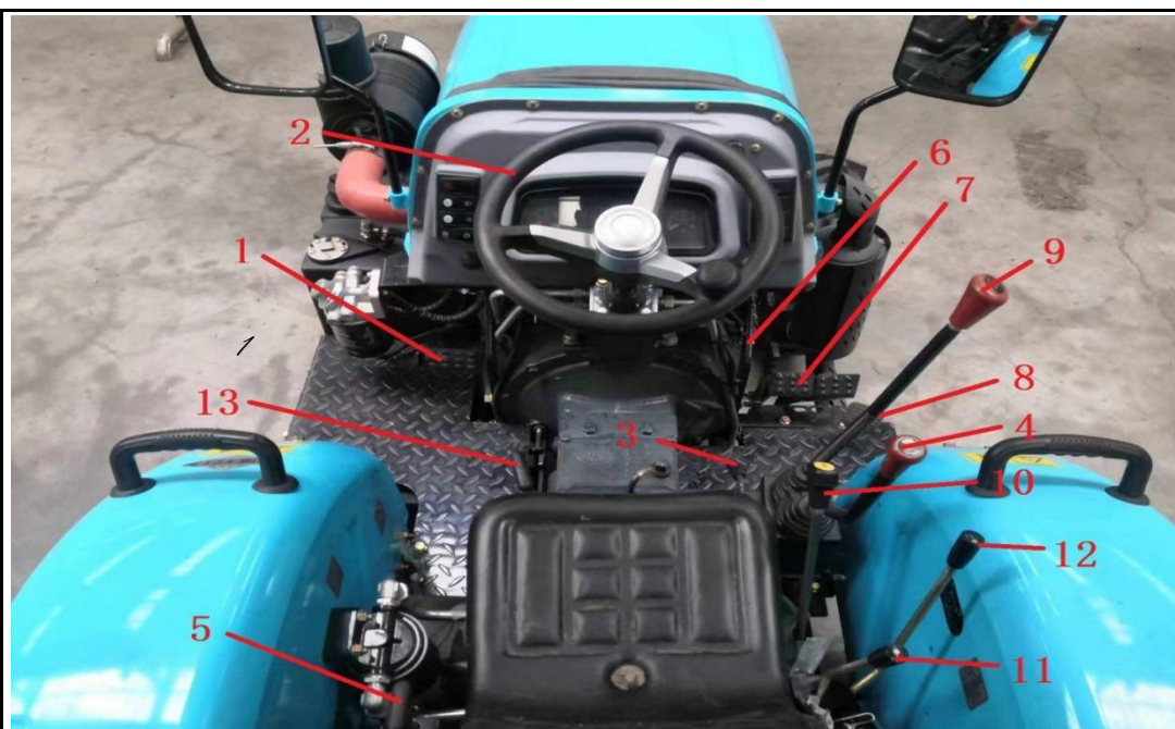
Mecanismo de control del tractor
