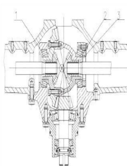
Ajuste del cojinete de la carcasa del diferencial
