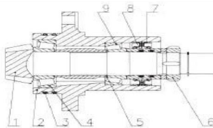
Ajuste de la transmisión central del eje motriz delantero
