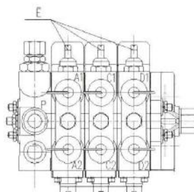
Figura 3-70 Salida hidráulica
