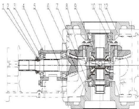
Figura 5-20 Transmisión central
