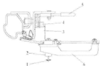
Figura 3-61 Mecanismo de puertas
