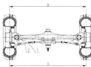
Figura 3-50 Eje motriz delantero
