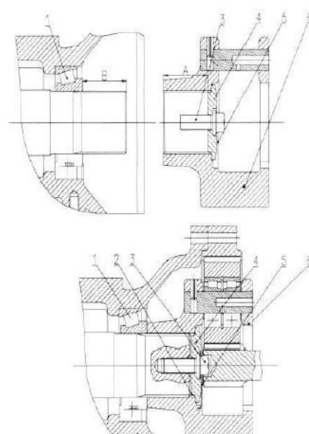
Figura 5-22 Transmisión final
