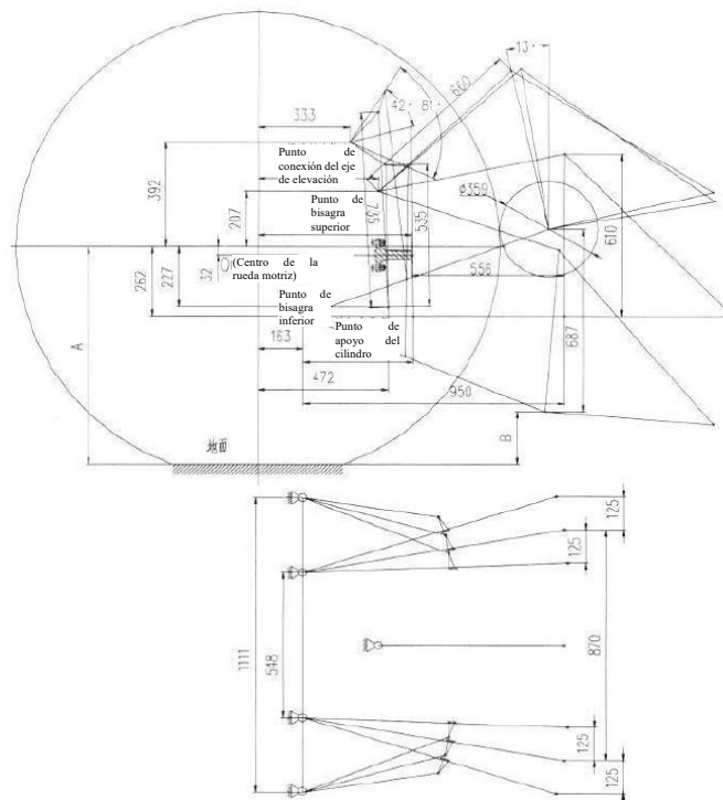
Figura 3-75 Plano de dimensiones del sistema de enganche
